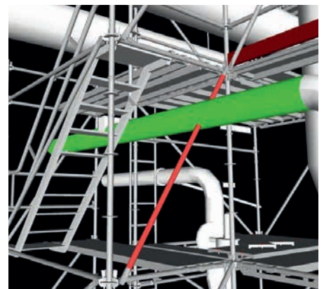
Kollisionsprüfung in Autodesk Navisworks Manage
