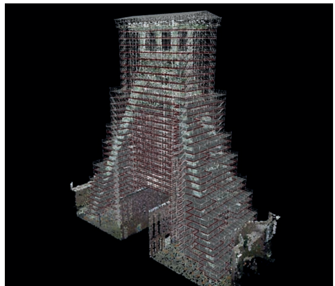
Punktwolke mit Gerüstplanung
