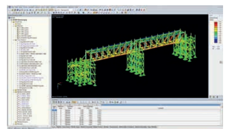
Statische Berechnung in RSTAB
