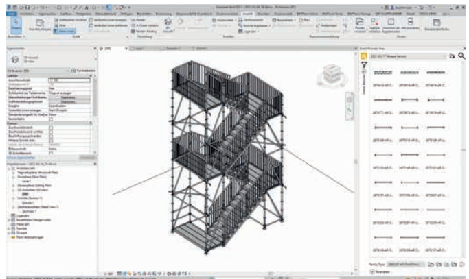
Planung einer Gerüstkonstruktion in Autodesk Revit
