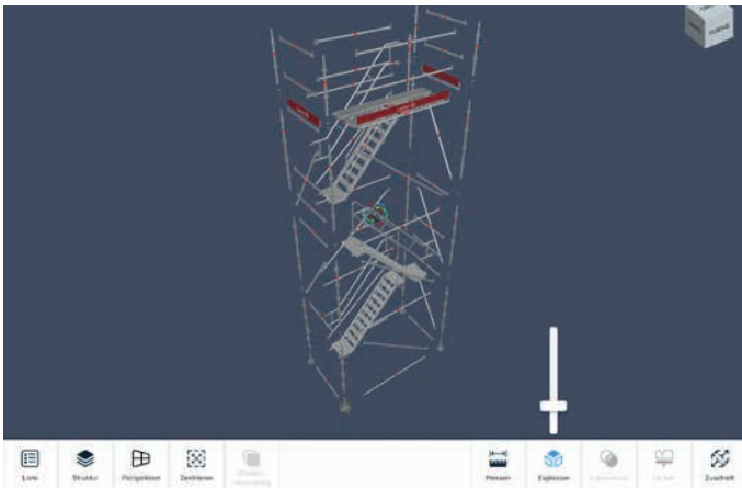
Explosions-Modus zur Darstellung von Details des Zusammenbaus
